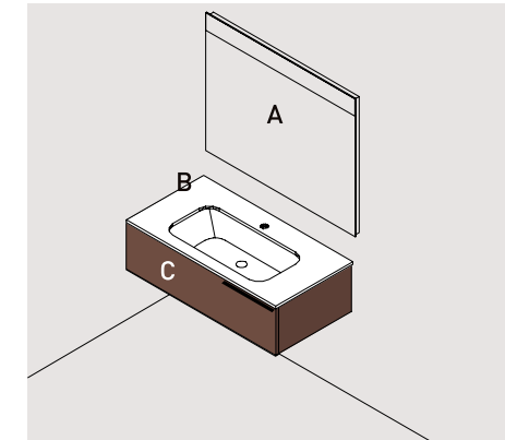
COMPOSIZIONE 90C3 L90 P46,5 cm
